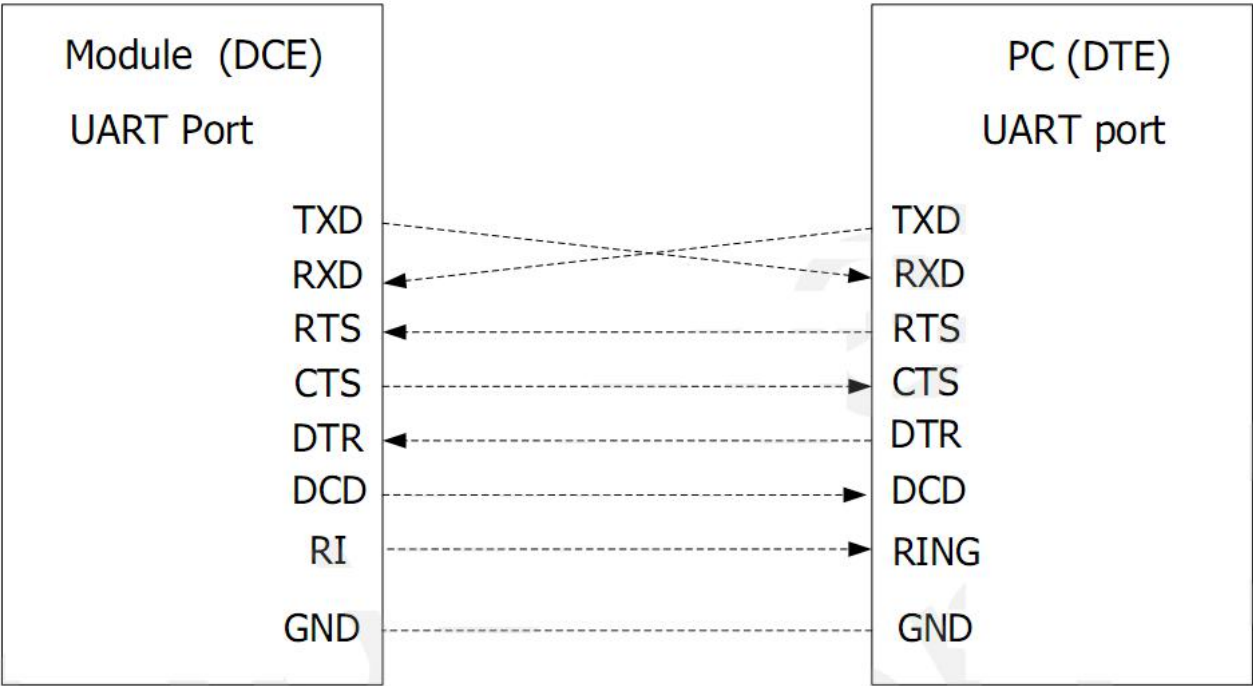
图 11：串口连接图
