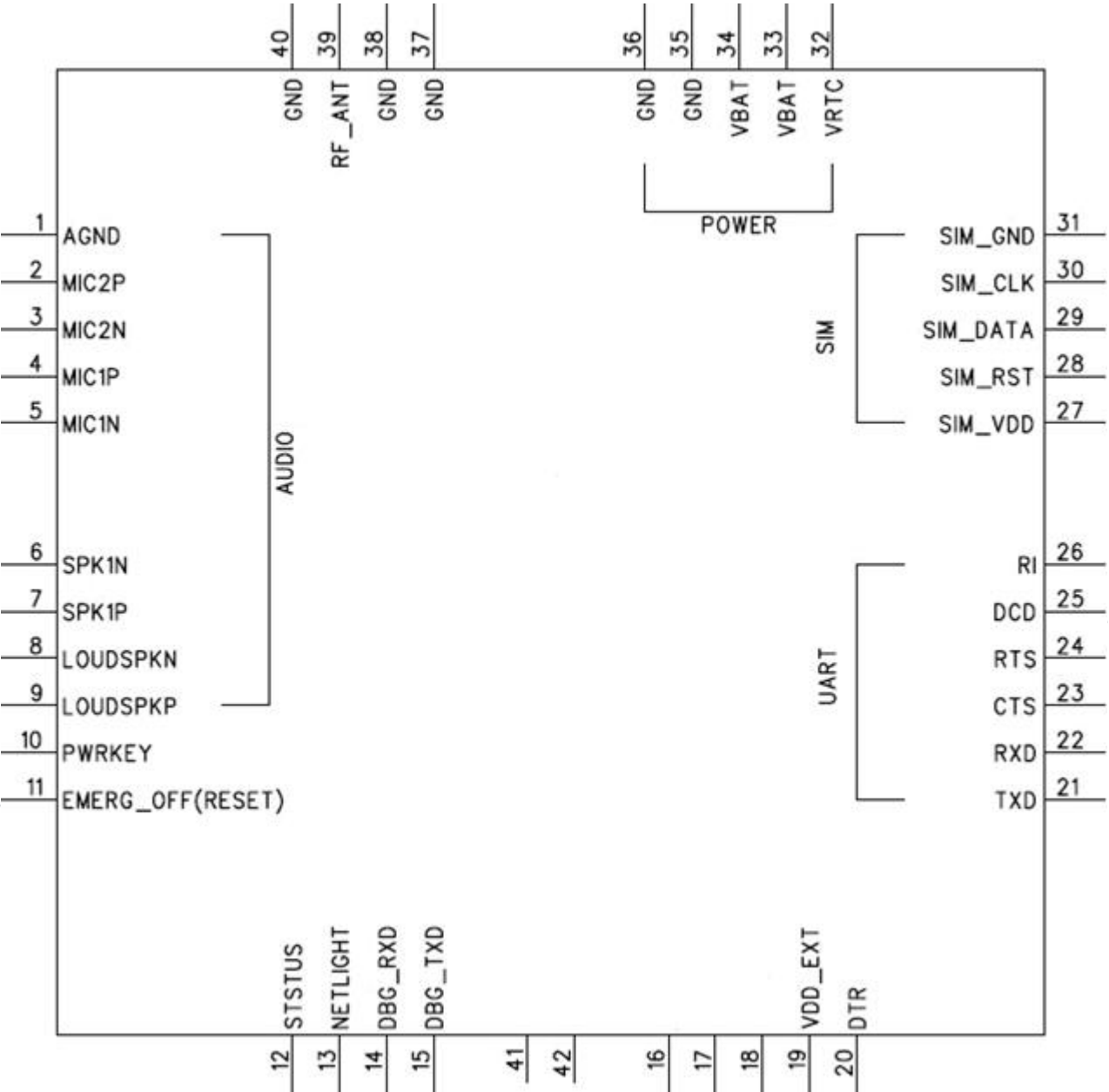
图 26: G3524 引脚图 (顶视图)
