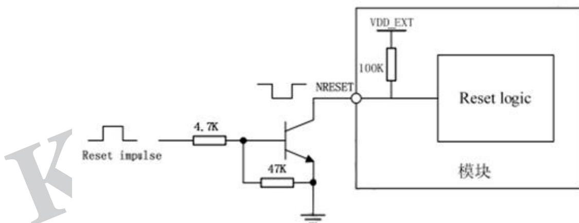
图 22：复位参考设计电路
