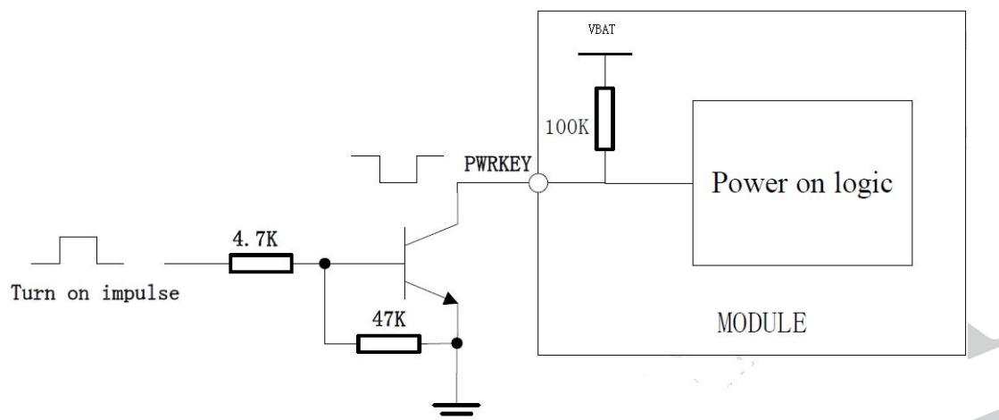
图 5：使用 PWRKEY 驱动电路开机
