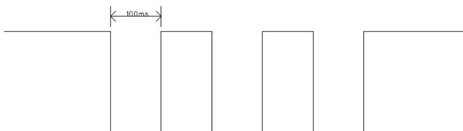
图 8：短信唤醒主控，RI 脚波形
