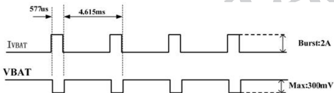
图 3: 突发时 VBAT 的跌落
