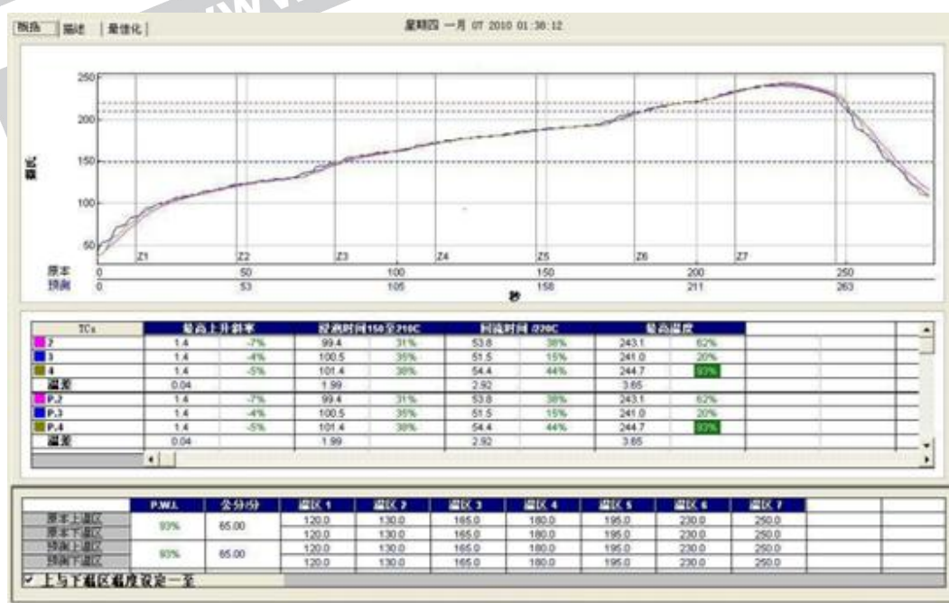
图 27: G3524 推荐焊接炉温曲线图
