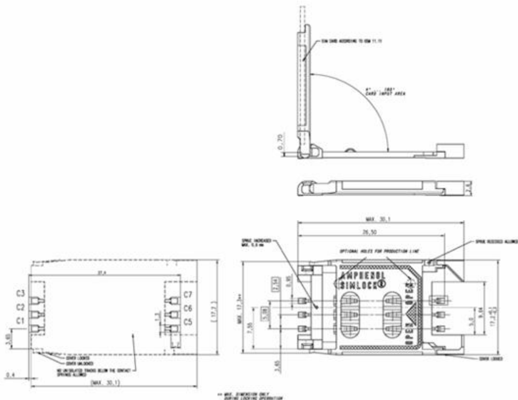
图 19: Amphenol C707 10M006 5122 SIM 卡座尺寸图
