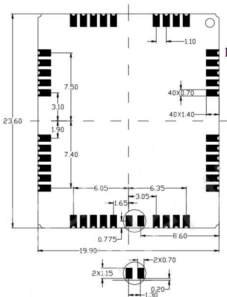
图 24: 模块俯视图的细节机械尺寸 (单位: mm)
