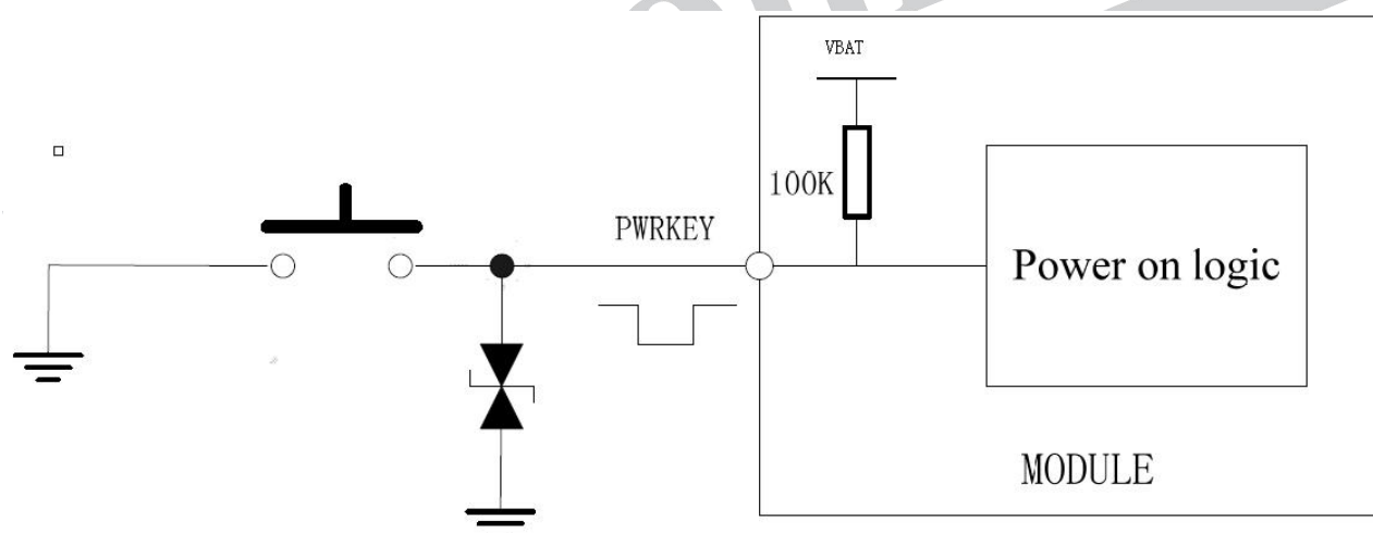
图 5：使用 PWRKEY 驱动电路开机
